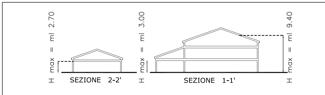
Scala 1:500
